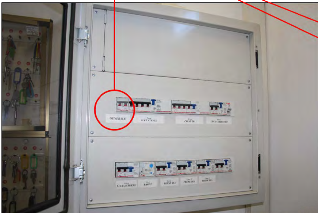
Quadro di zona 1 Piano Primo
