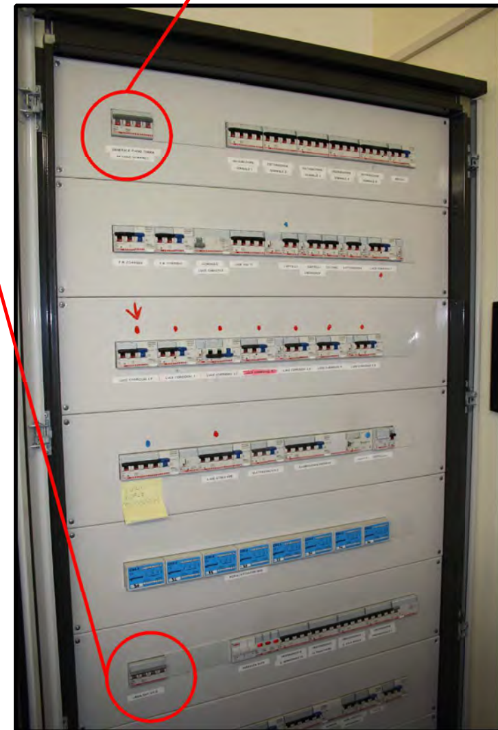
Quadro Elettrico Piano Terra
