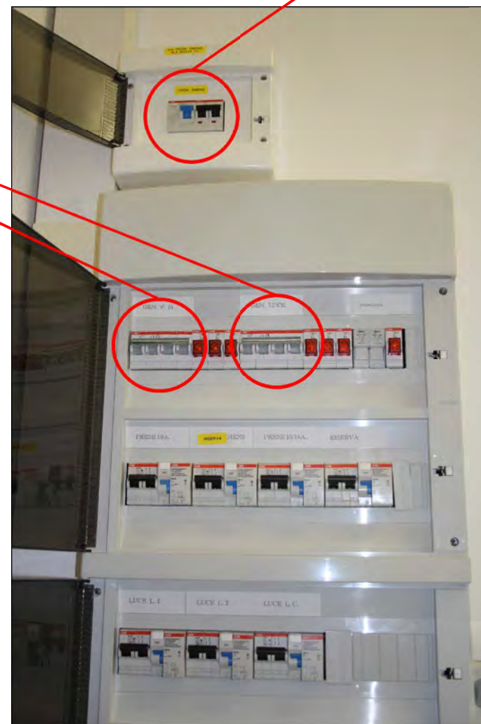
Quadro di zona 2 Piano Primo
