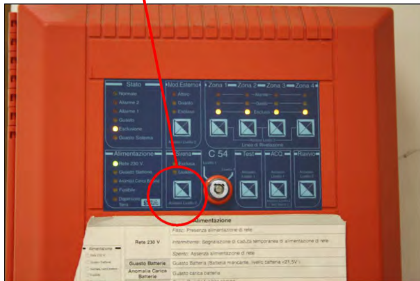
Centrale Rilevazione Incendi
